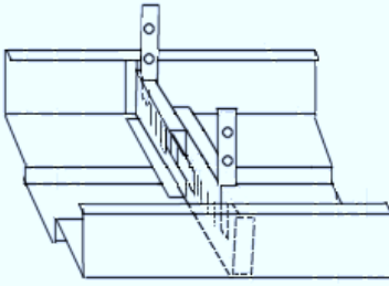
drywall (DW)
