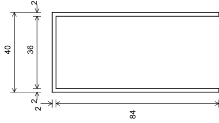
Elev A
